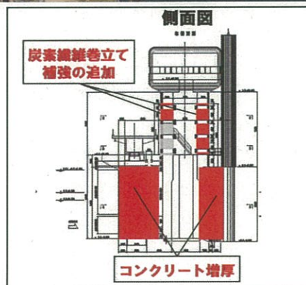
堰柱耐震補強図
