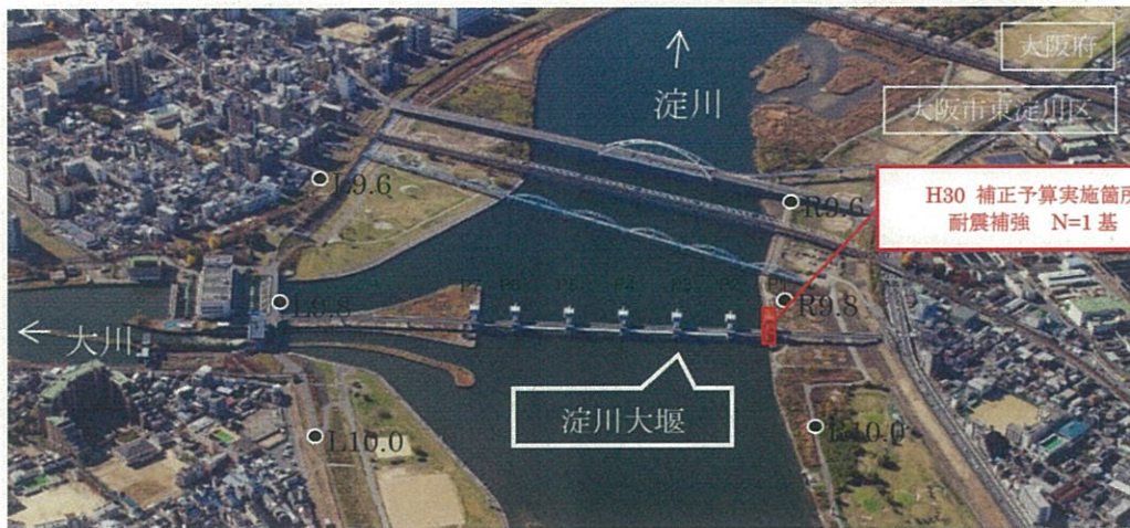
堰柱耐震補強図
